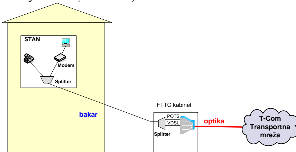
30. Način realizacije FTTC koncepta u pristupnoj mreži
