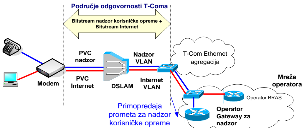
Slika 29. Veleprodajni širokopoljasni pristup za pružanje usluge nadzora korisničke opreme preko ADSL/VDSL pristupa na DSLAM razini
